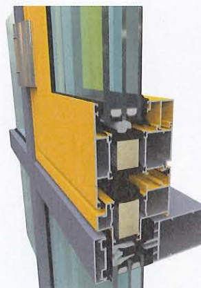
Mit dem Fenstersystem AT 740 SI können nach außen öffnende Fenstervarianten montiert werden.
